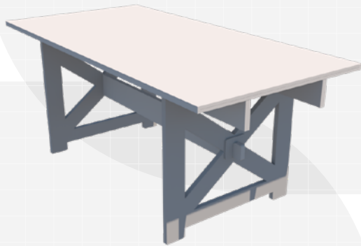
TA-020 Picnic Table 01 - 72" 72" (W) x 36" (D) x 30" (H)
